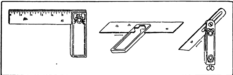
Fig. 200. Try-Square.
