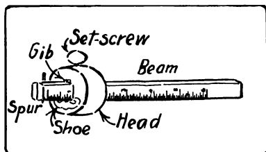
Fig. 211. Marking-Gage.
