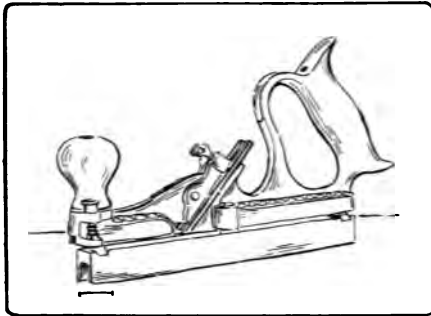
Fig. 115. Tonguing-and-Grooving-Plane.
