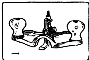
Fig. 121. Router-Plane.
