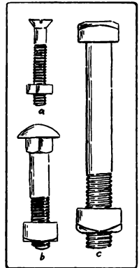
Fig. 230. a. Stove-bolt. b. Carriage-bolt. c. Machine-bolt.
