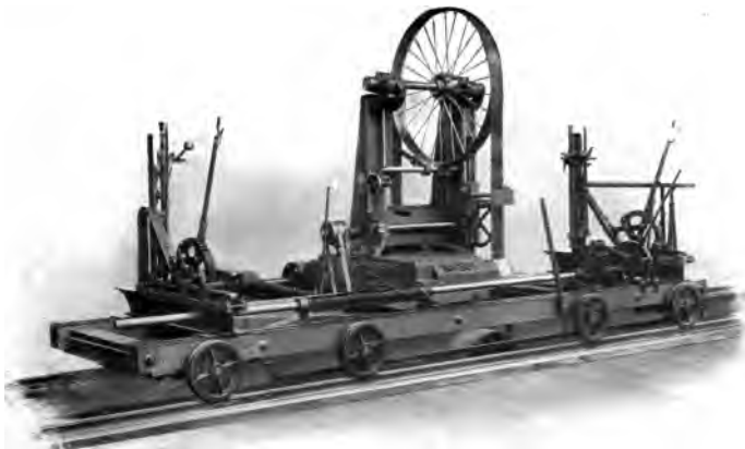
Fig. 34. Band-Saw.
