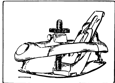
Fig. 116. Circular-Plane.
