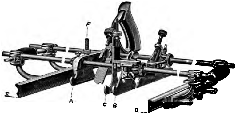
Fig. 117. Universal Plane.
